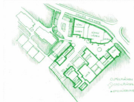
Brennerei Elmendorf - Lageplan / Nutzung - Bauplanarchitekten 20.02.04
